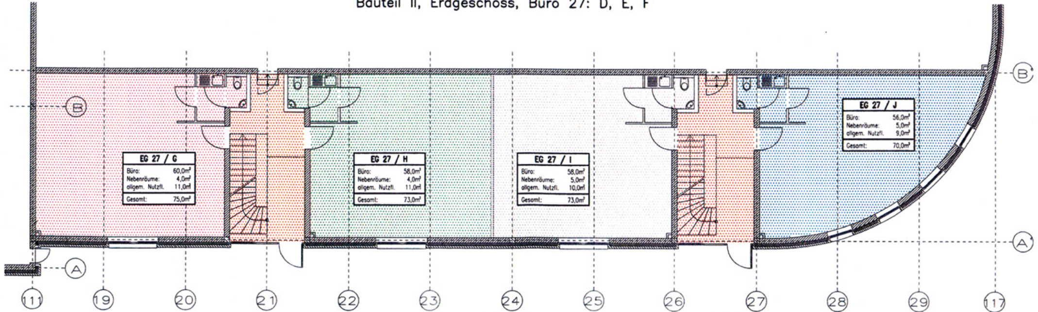
Bauteil III, Erdgeschoss, Büro 27: G, H, I, J
