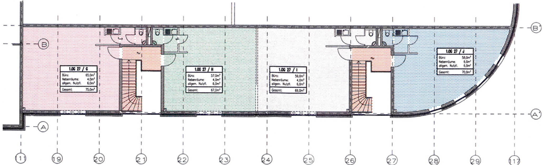
Bauteil III, 1. Obergeschoss, Büro 27: G, H, I, J
