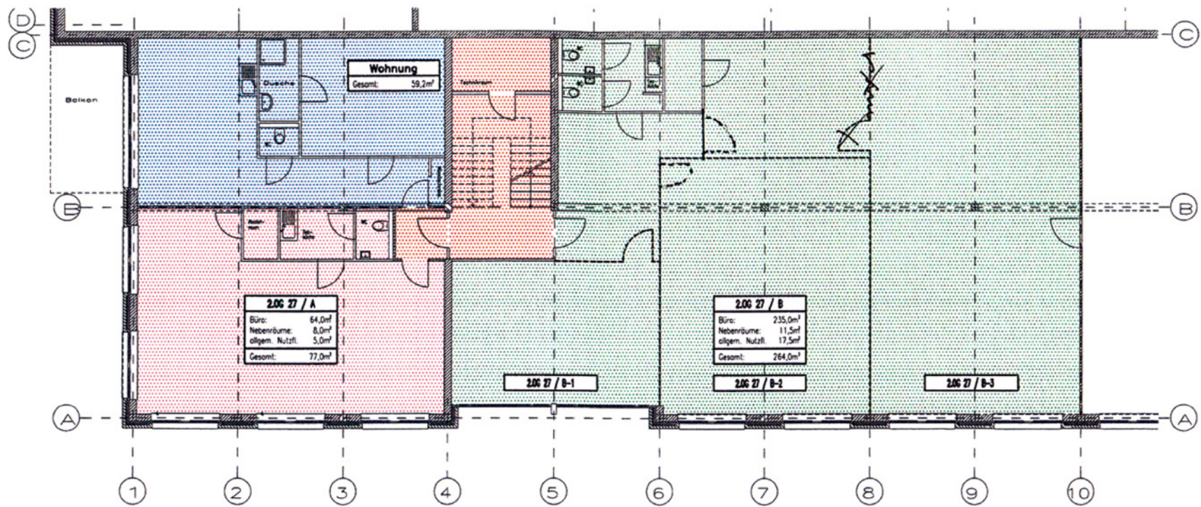
Bauteil I, 2. Obergeschoss, Büro 27: A, B
