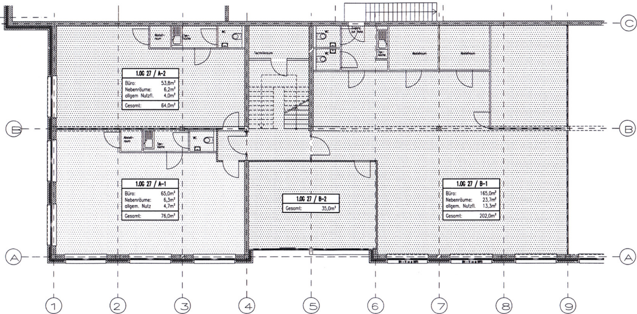
Bauteil I, 1. Obergeschoss, Büro 27: A-1, A-2, B-1, B-2
